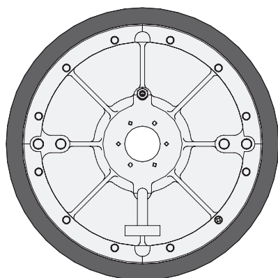
66516-X 顶视图 (显示螺栓的布局)
