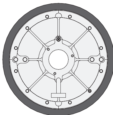
66517-X 顶视图 (显示螺栓的布局)
